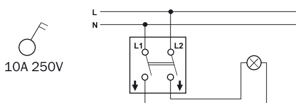
Одноклавишный выключатель двухполюсной
