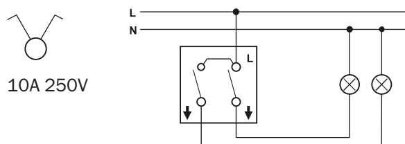
Двухклавишный выключатель
