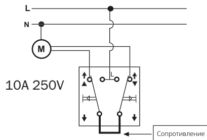
Проходной кнопочный переключатель для жалюзи (управление с 1 места)
