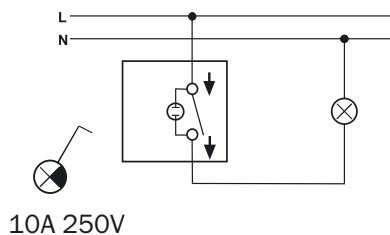
Одноклавишный выключатель с подсветкой
