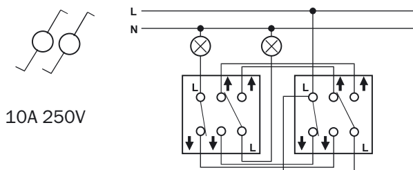
Двухклавишный проходной выключатель
