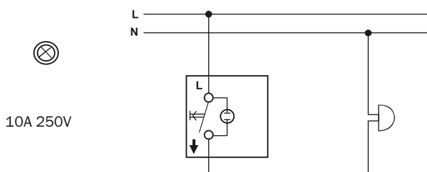
Кнопочный выключатель с подсветкой (250V)
