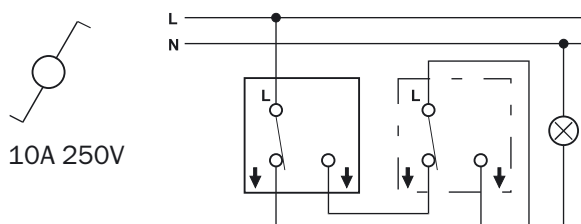
Проходной выключатель с 2-х мест
