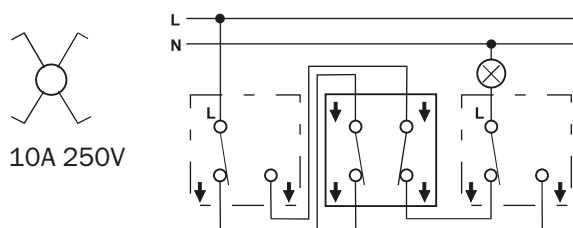
Проходной выключатель
