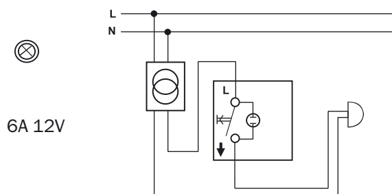
Кнопочный выключатель с подсветкой (12V)
