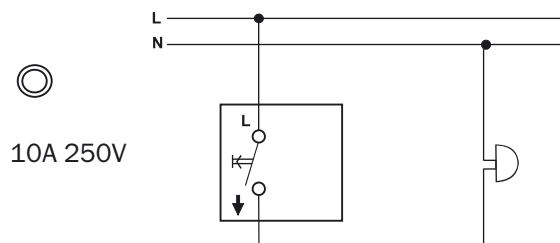
Кнопочный выключатель
