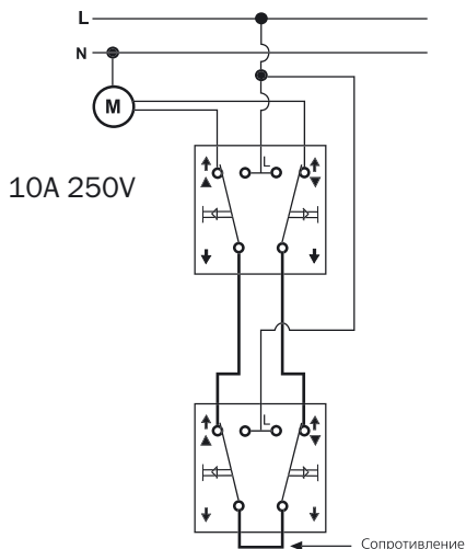
Проходной кнопочный переключатель для жалюзи (управление с 2-х мест и более)
