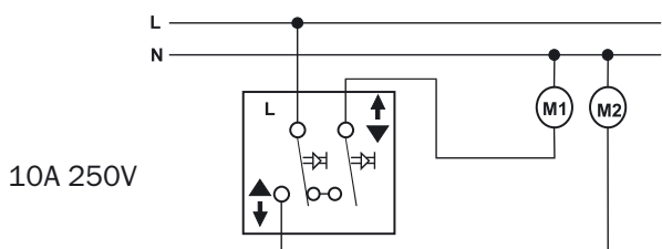
Поворотный переключатель
