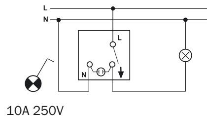
Одноклавишный выключатель с сигнальной лампой
