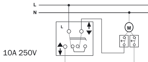
Выключатель для жалюзи
