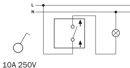
Одноклавишный выключатель
