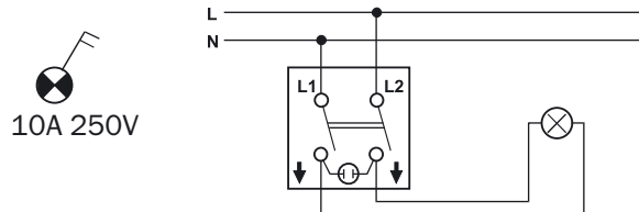
Одноклавишный выключатель двухполюсной с сигнальной лампой
