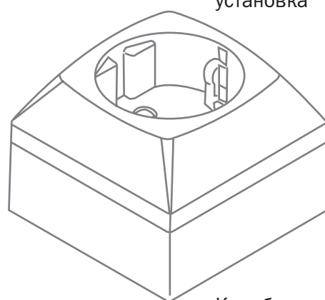
Коробка для установки изделия серии 47 без миниканала
