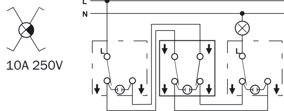
Проходной выключатель с подсветкой
