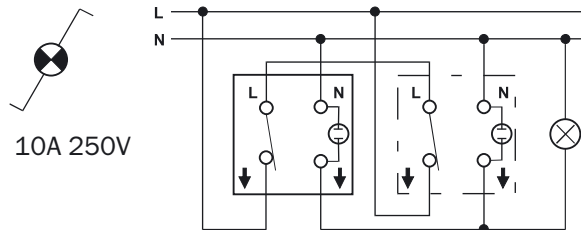
Проходной выключатель с 2-х мест с подсветкой
