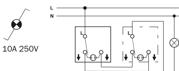
Проходной выключатель с 2-х мест с сигнальной лампой
